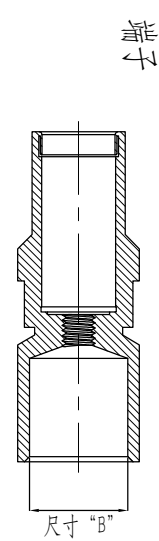
剖面视图 B-B 1:1
